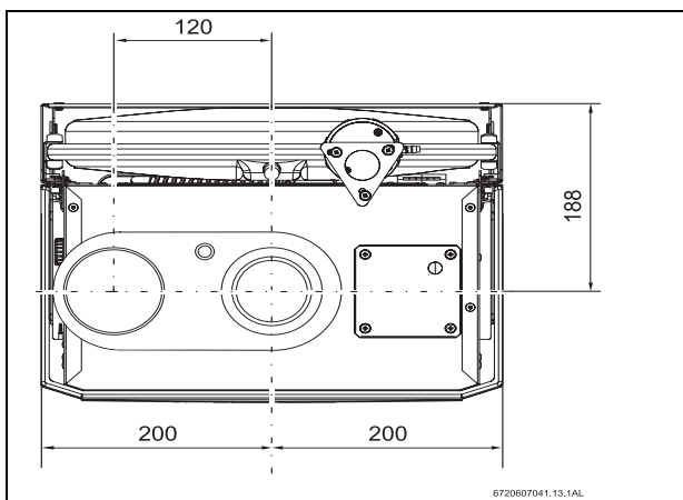
Fig. 2 Vista dall'alto con sdoppiatore 80/80 mm (acc. AZ 377)
