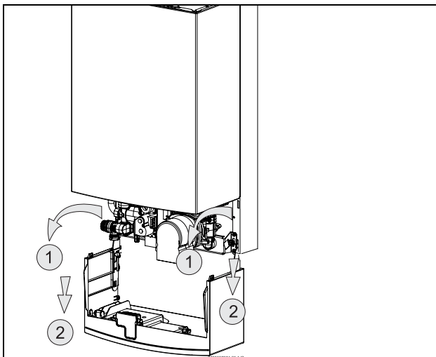
Fig. 24 Posizione di manutenzione per l'accesso ai componenti
