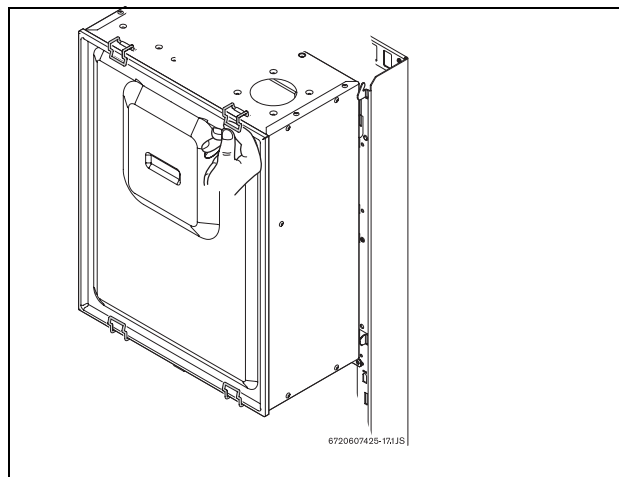
Fig. 22 Coperchio stagno della camera combustione
