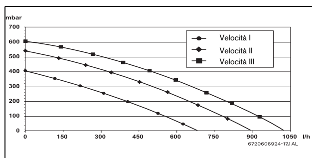
Fig. 5 Curva caratteristica del circolatore
